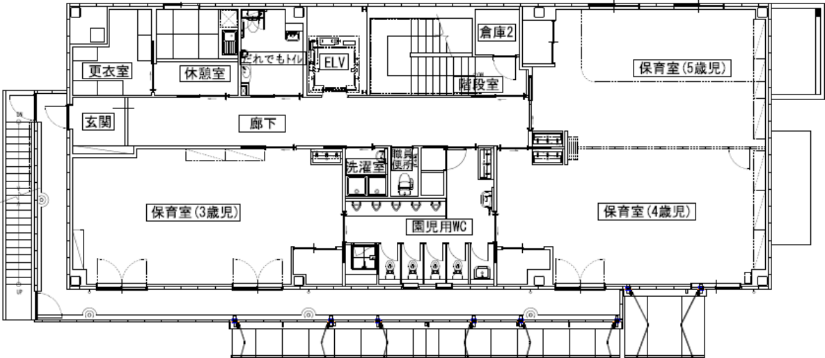
2F平面図
